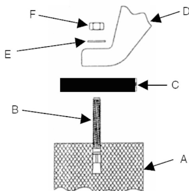
Montage-type
